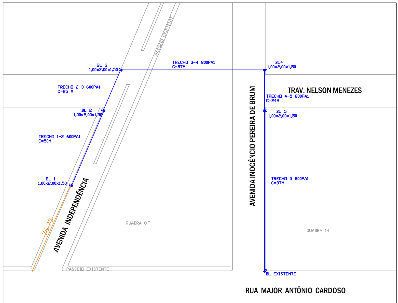
Escala: 1/100
